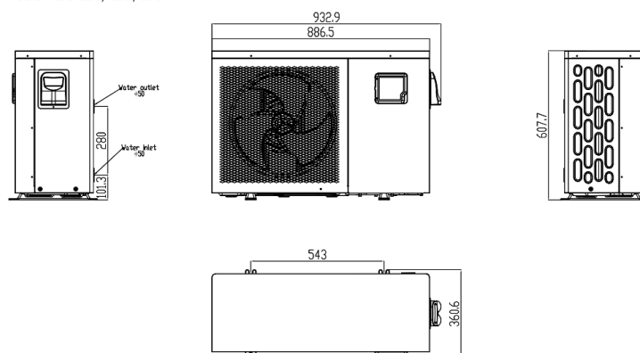
Model : DC E35/E55/E75
